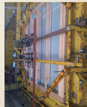
● 第三者機関での「耐風圧性能試験」の様子
