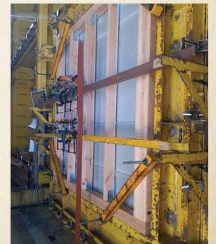
● 第三者機関での「耐風圧性能試験」の様子
