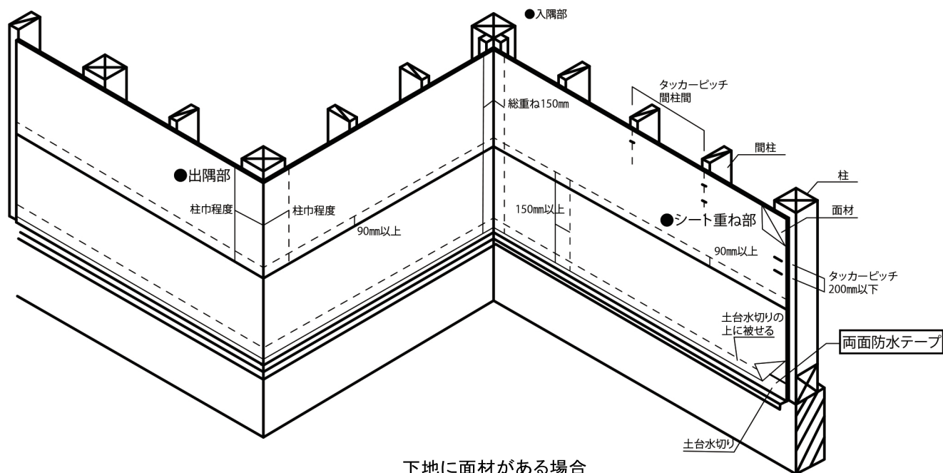
下地に面材がある場合
